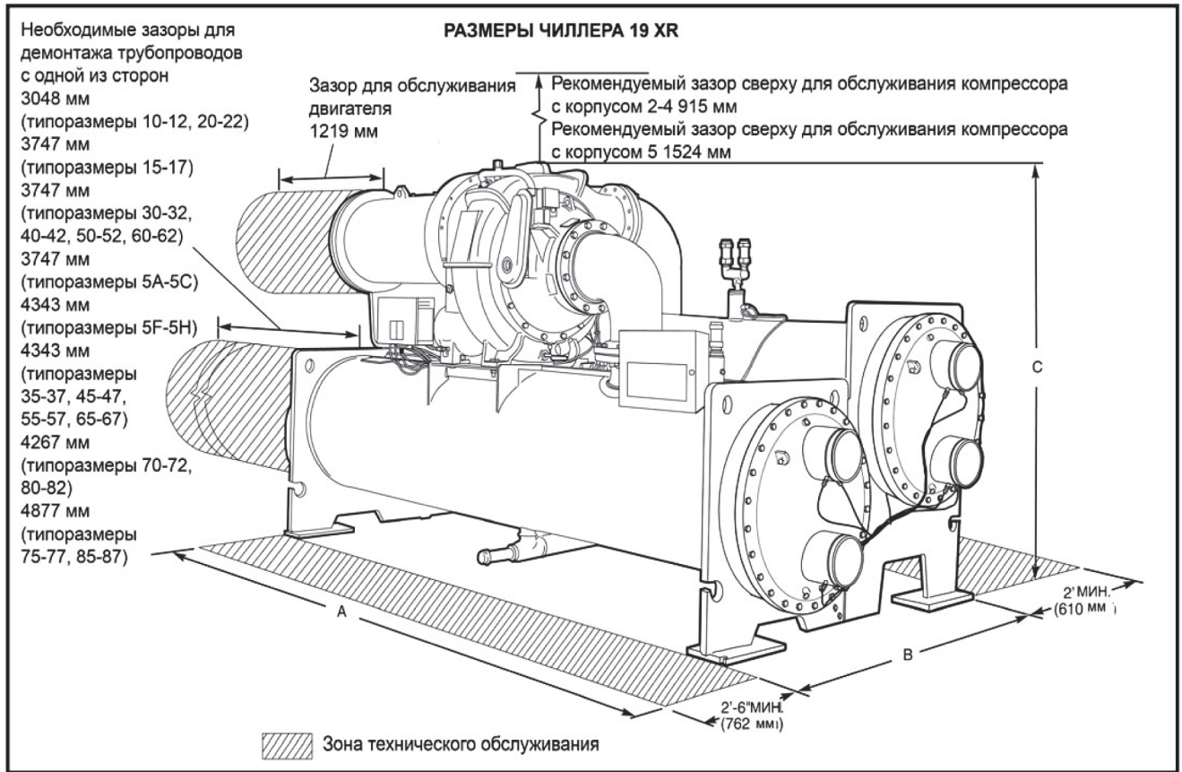
Размеры 19 XR (судовая водяная камера)
