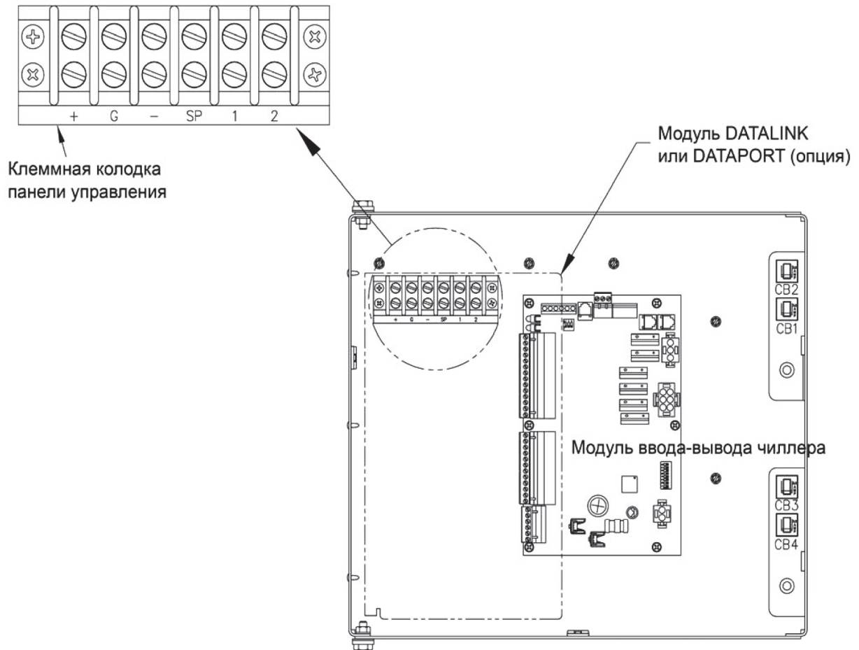
РАСПОЛОЖЕНИЕ КОМПОНЕНТОВ ПАНЕЛИ УПРАВЛЕНИЯ
