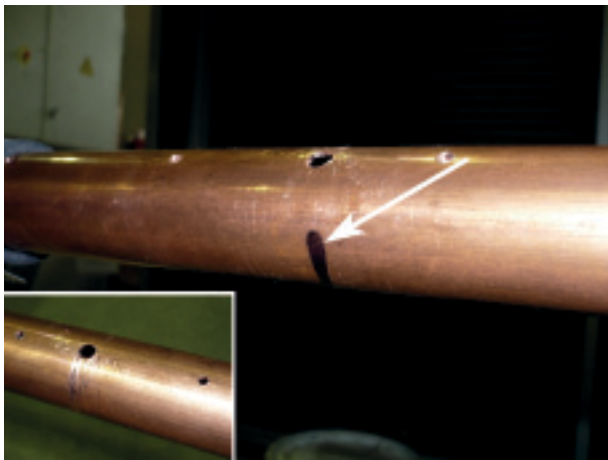
Установочное отверстие
