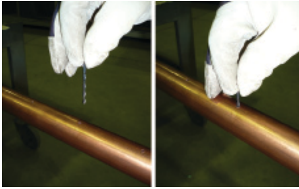
Прочистка оросительных отверстий
