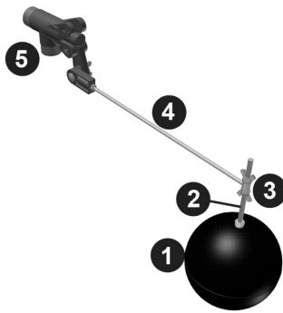
Узел клапана подпитки водой
