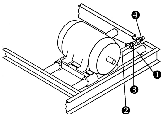
Регулируемое основание мотора
