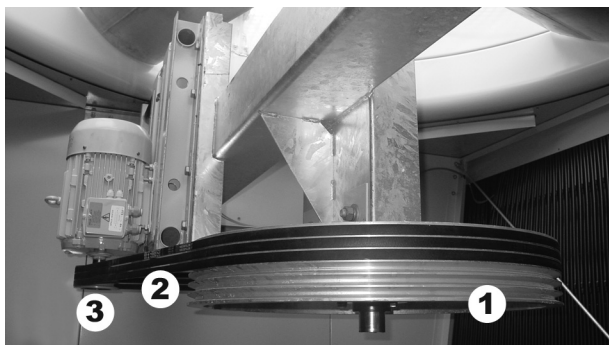
Ременный привод
