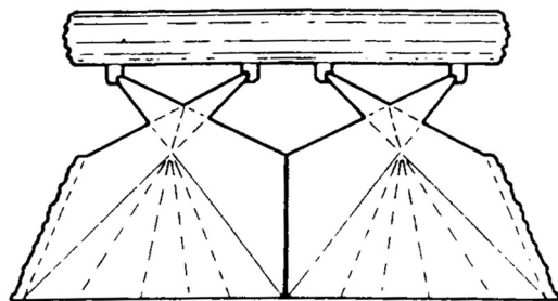
Структура разбрызгивания форсунок для грядирни
