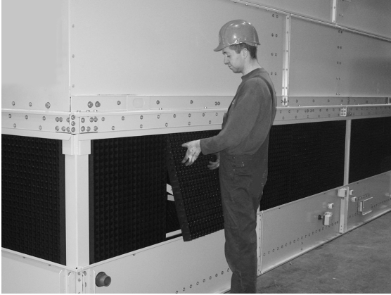
Снятие комбинированных экранов на входе
